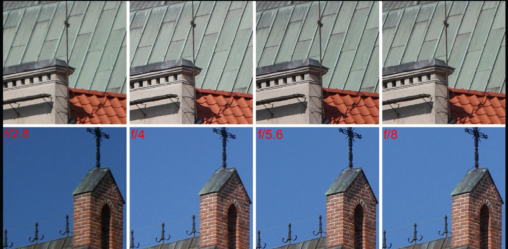
Wycinki ze zdjęć z telezooma, z centrum kadru (górne) i z obrzeża (dolne) dla czterech otworów przysłon i ogniskowej 100 mm.
