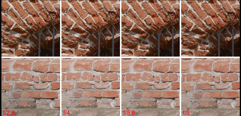
Wycinki ze zdjęć z zooma standardowego, z centrum kadru (górne) i z obrzeża (dolne) dla czterech otworów przyston i ogniskowej 12 mm.
